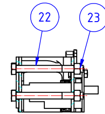
A-A (1:2)
